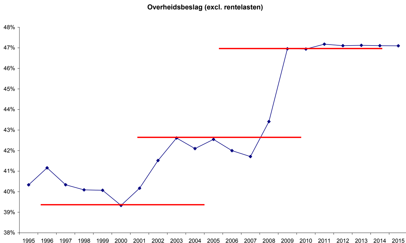
Grafiek 1: Overheidsbeslag (excl. rentelasten): % BBP
